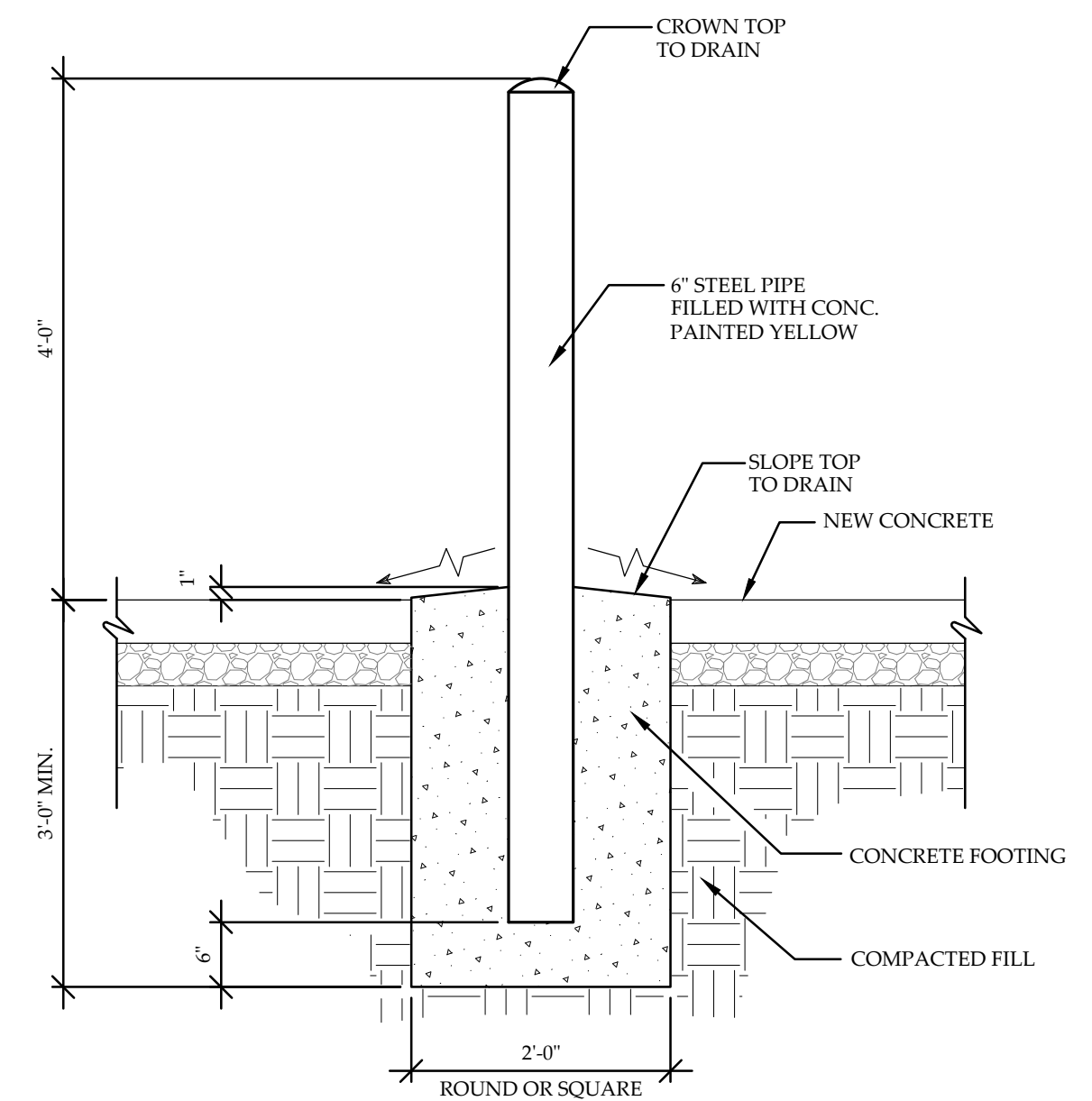
B BOLLARD DETAIL SCALE: 3/4"=1'-0"
