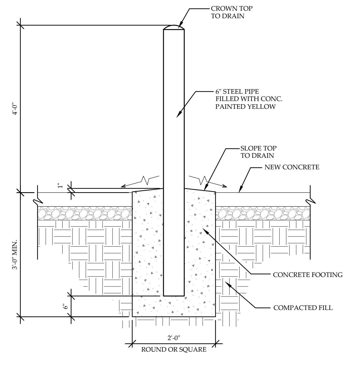
B BOLLARD DETAIL SCALE: 3/4"=1'-0"
